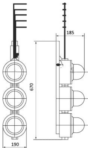
Рис. 1 Указатель троллейный К-271 У2 металлический
