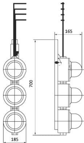
Рис. 2 Указатель троллейный К-271Н У2 полиамид
